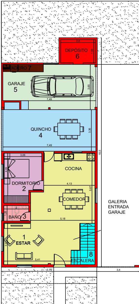
PLANTA BAJA
